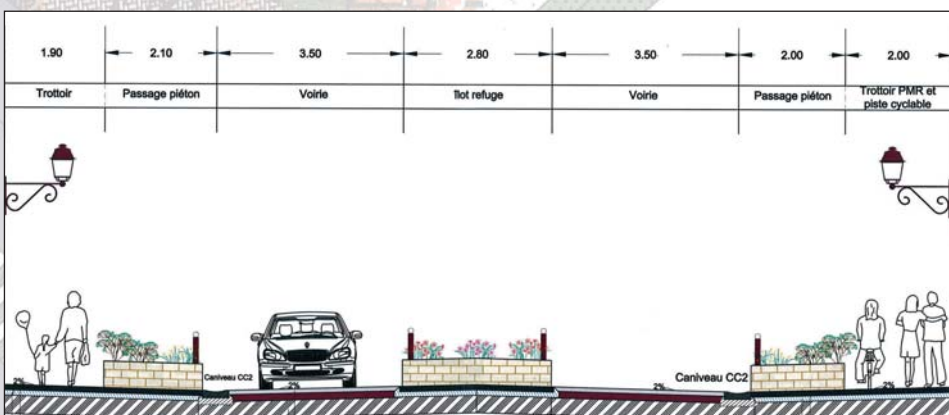
Coupe transversale présentant un exemple d'aménagement d'une section de la rue de Flamanville.
